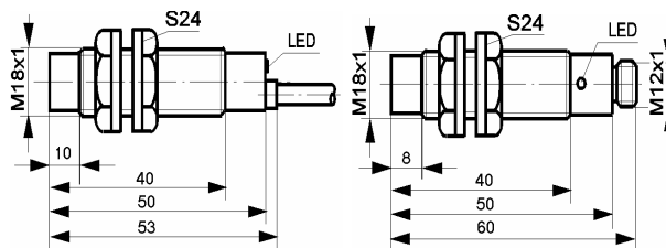
wyjście kablowe
