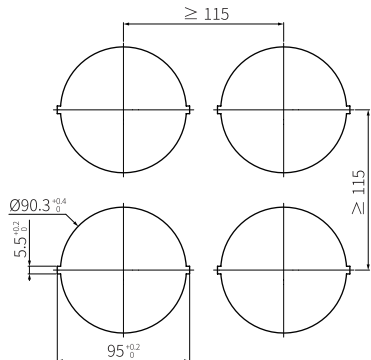
• 齐平型保护罩面板加工尺寸图
