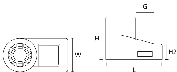
Cable tie base CTMS5
