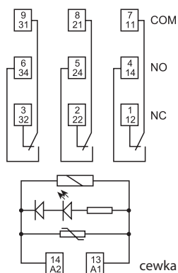
Przykład: AC
