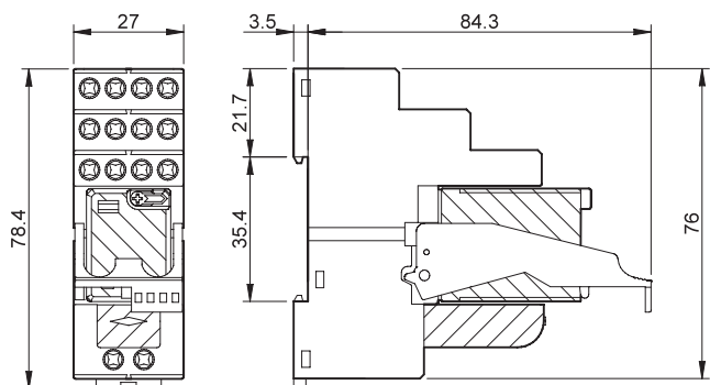
Typ 58.P3 Zaciski Push-in
