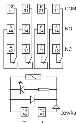
Przykład: DC
