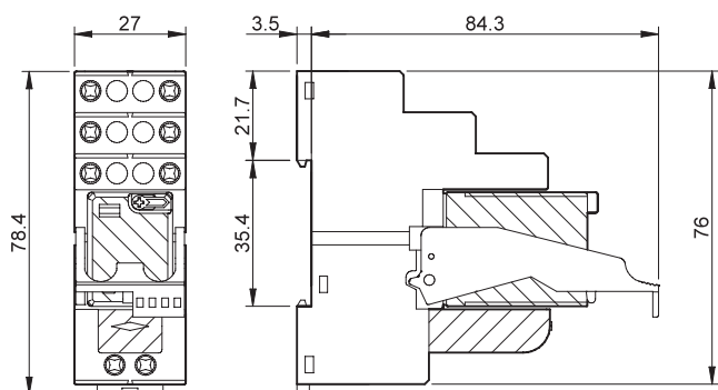
Typ 58.34 Zaciski śrubowe
