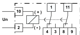
Schemat wyprowadzeń
