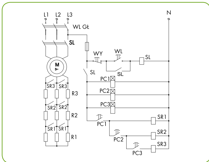
Przykład 1: Układ rozruchowy silnika indukcyjnego pierścieniowego.
