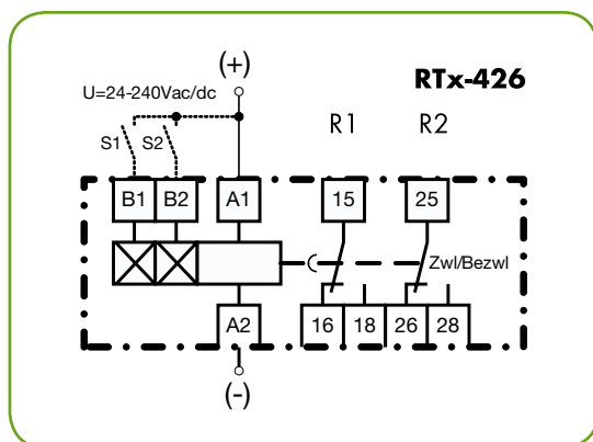
Schemat wyprowadzeń
