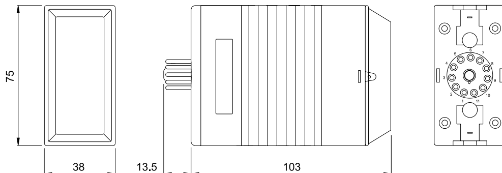
Wymiary przełącznika: RTox-10
