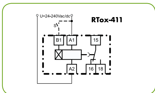
Schemat wyprawdzeń
