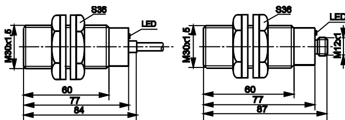
wyjście kablowe
