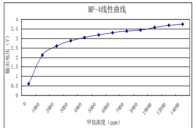
Linear curve
