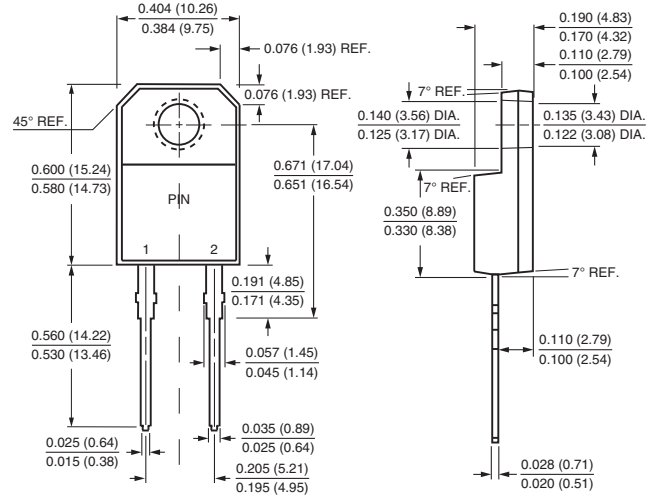
ITO-220AC
