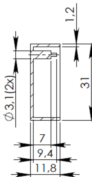
PRZEKRÓJ A-A
