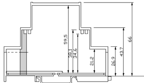
BARRA DIN
