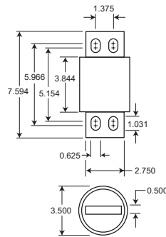
Fig. 2: 900-1000 Amp Range
