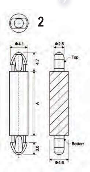
Obere & Untere Bohrung \varnothing 3.5 \pm 0.05 mm Obere Platten Stärke 1.57 mm Typ 2
