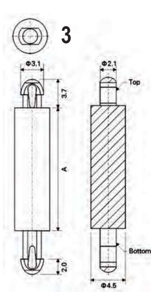
Obere & Untere Bohrung \varnothing 2.5 \pm 0.05 mm Obere Platten Stärke 1.57 mm Untere Platten Stärke 3.6 mm Typ 3
