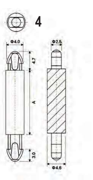
Obere & Untere Bohrung \varnothing 3.5 \pm 0.05 mm Obere Platten Stärke 1.57 mm Untere Platten Stärke 3.6 mm Typ 4
