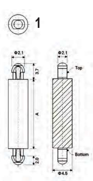
Obere & Untere Bohrung \varnothing 2.5 \pm 0.05 mm Obere & Untere Platten Stärke 1.57 mm Typ 1
