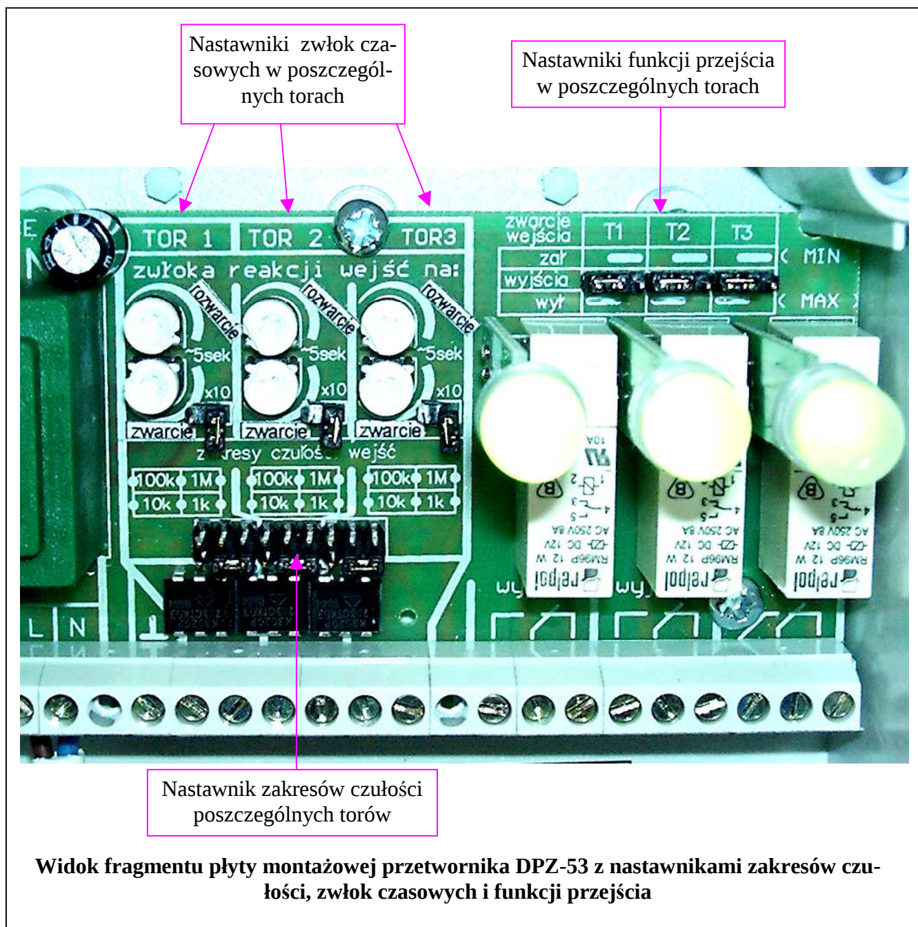
Rys. 6 Widok nastawników na płycie montażowej przetwornika DPZ-53
