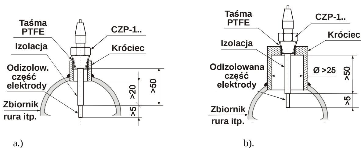
Rys. 5 Przykłady poprawnego montażu czujników
