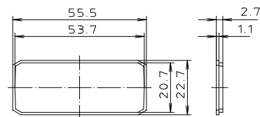
Frontplatte Kunststoff
