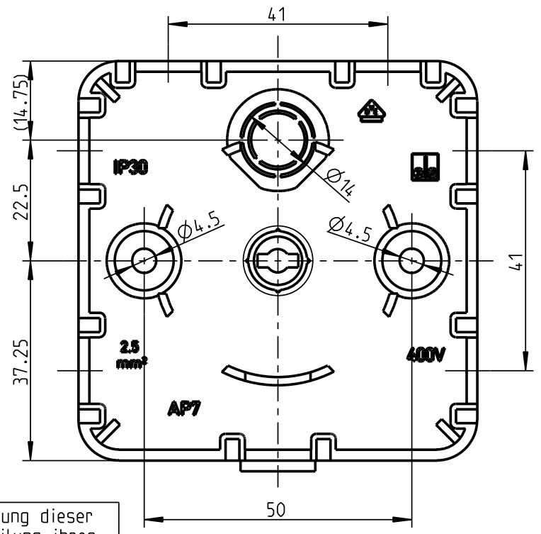
Innenansicht Unterteil
