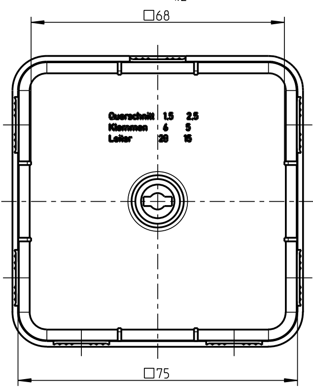
Innenansicht Deckel
