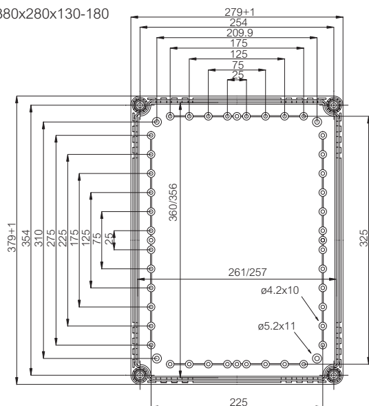
EK 380x280x130-180
