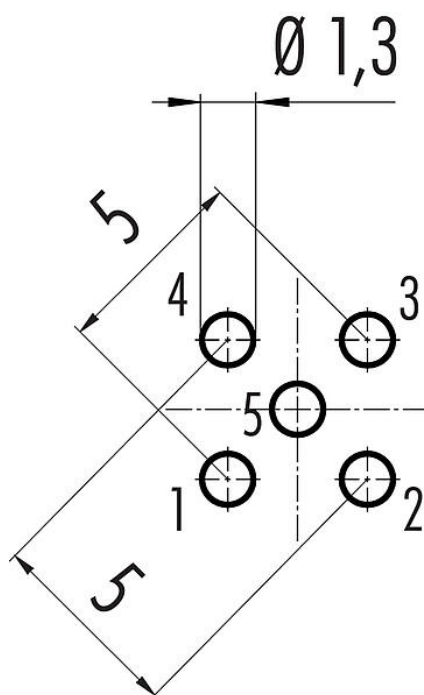
Układ przewodów
