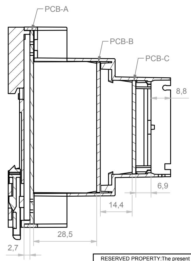
A-A (1:1)
