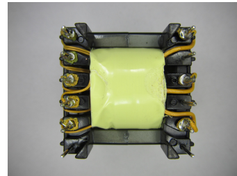
Zdjęcie transformatora
